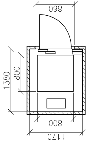
ПЛАН СПИРКА М 1:50
