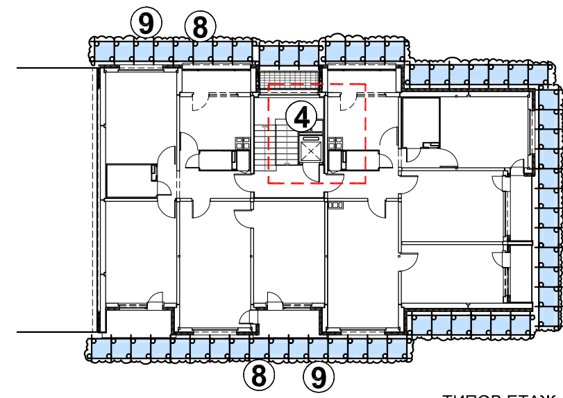
ТИПОВ ЕТАЖ
