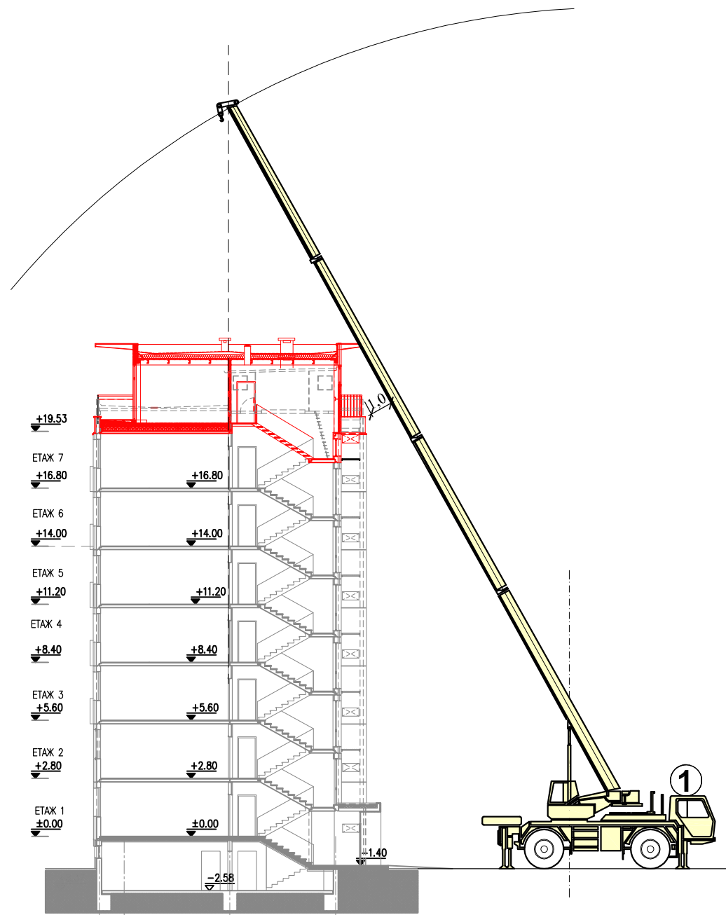
РАЗРЕЗ А-А
