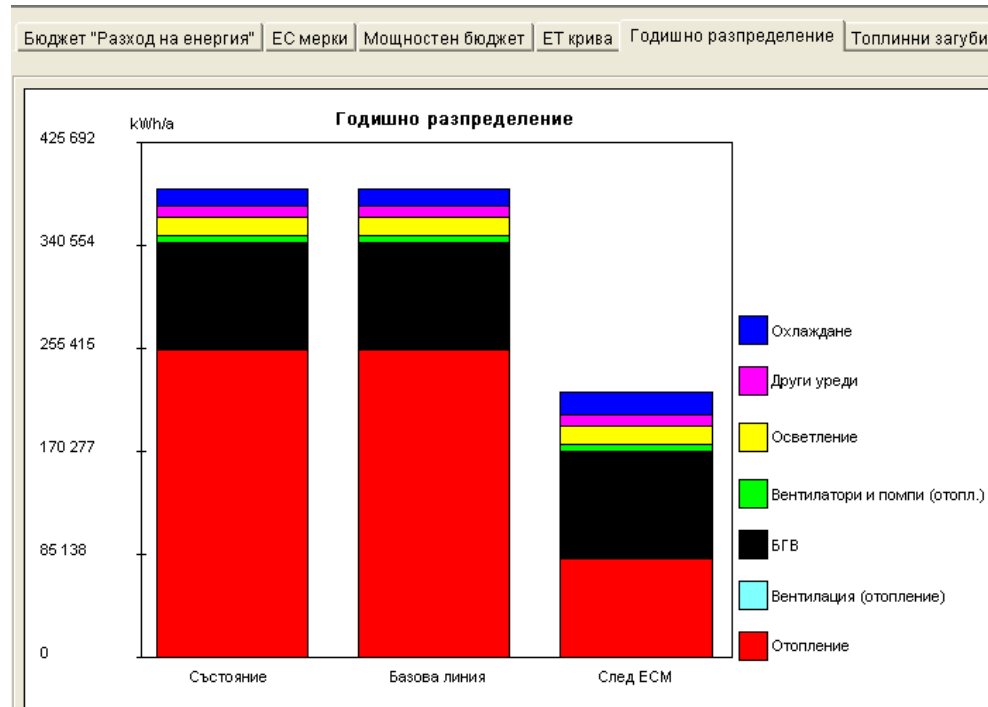
фигура 4 Годишно разпределение на разхода на енергия
