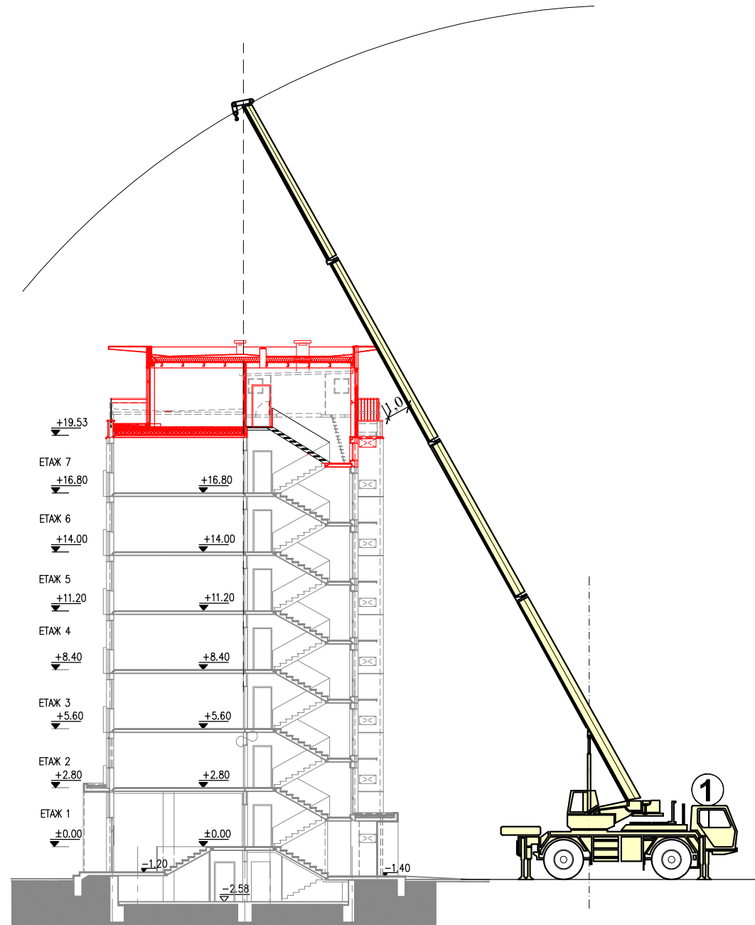
РАЗРЕЗ А-А
