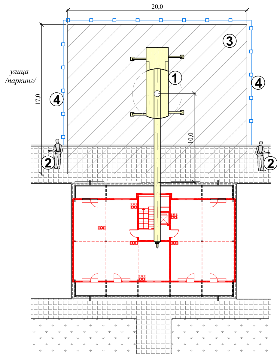
НАДСТРОЙКА МОНТАЖ НА ПАНЕЛИ ТИП "СПИРОЛ" И МЕТАЛНИ КОНСТРУКЦИИ
