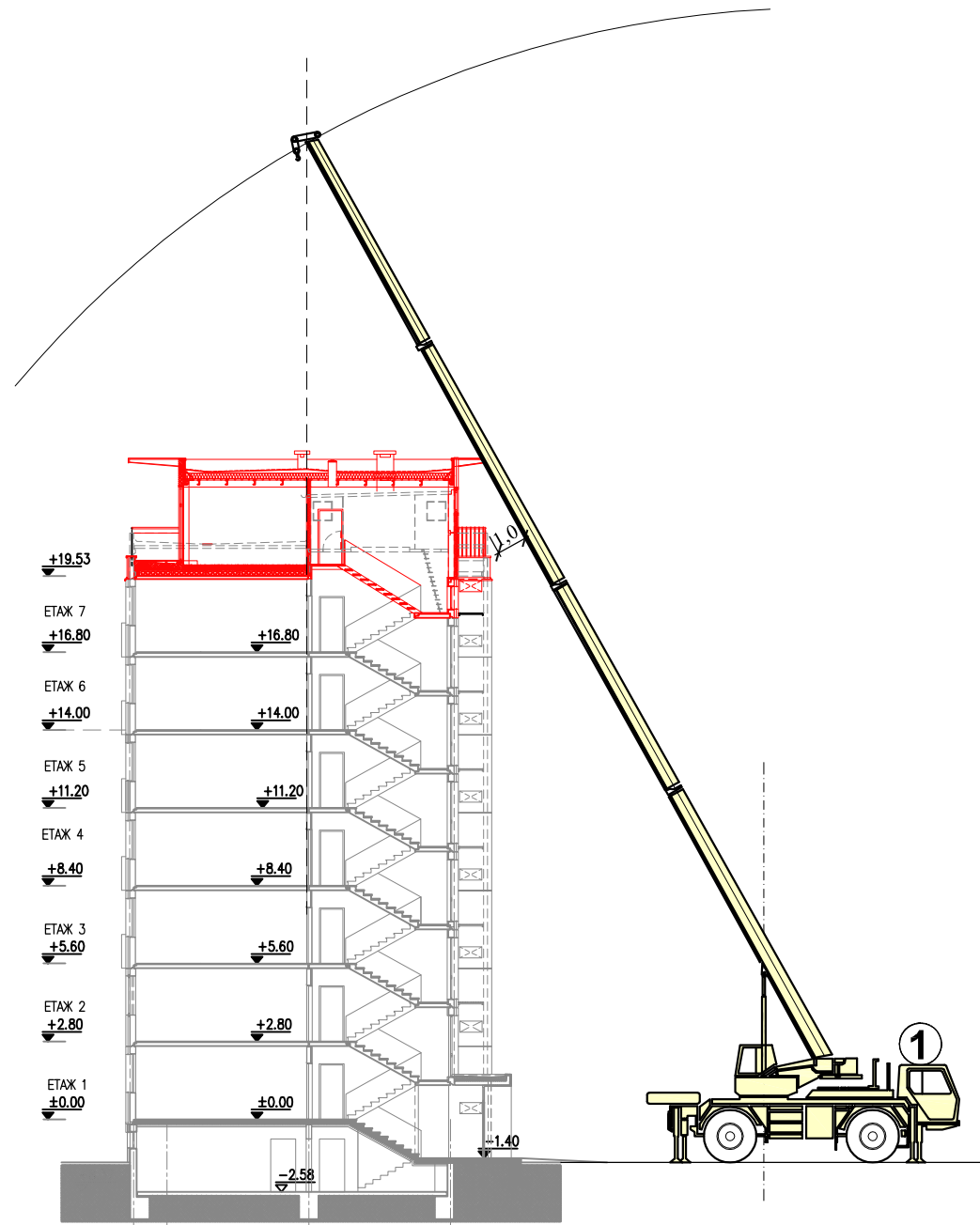
РАЗРЕЗ А-А
