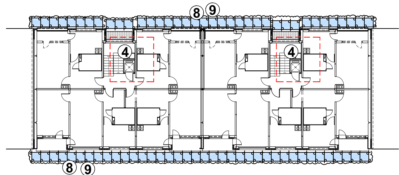
ТИПОВ ЕТАЖ
