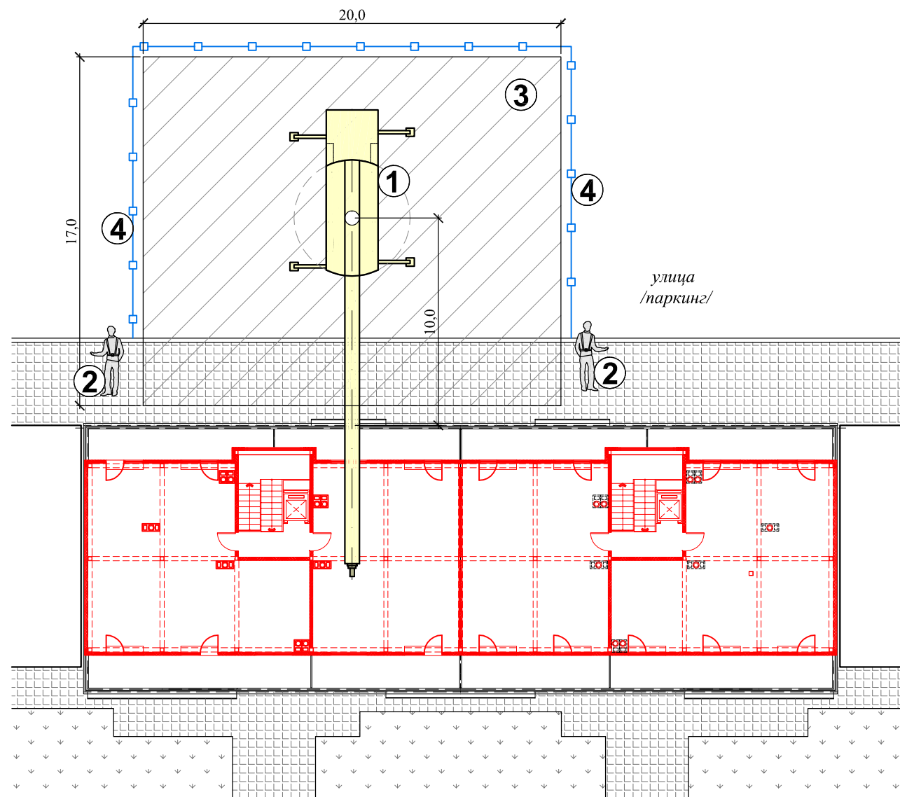
НАДСТРОЙКА МОНТАЖ НА ПАНЕЛИ ТИП "СПИРОЛ" И МЕТАЛНИ КОНСТРУКЦИИ
