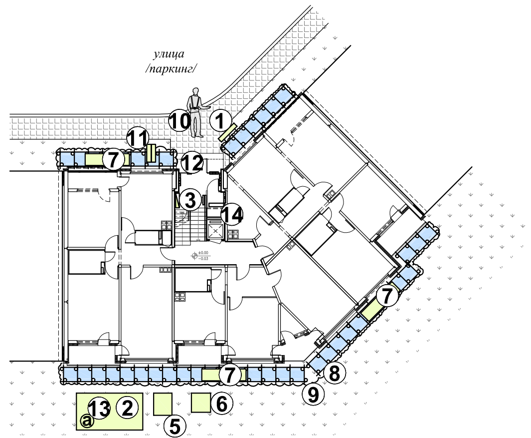
ПЪРВИ ЕТАЖ
