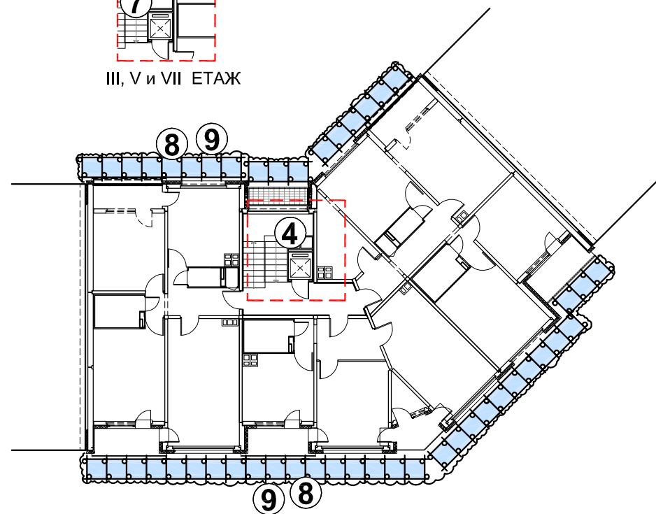
ТИПОВ ЕТАЖ
