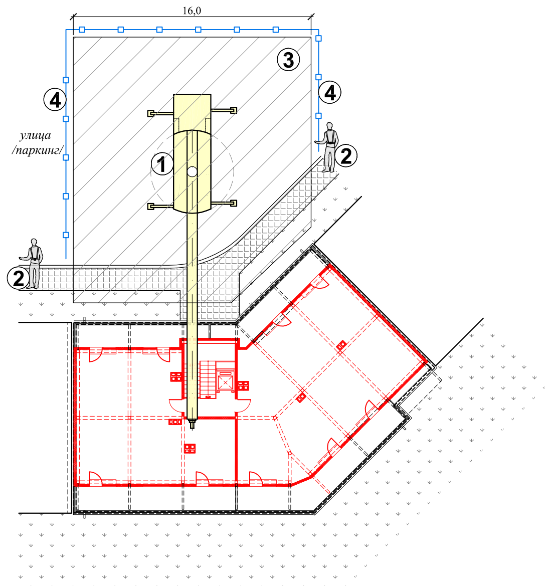
НАДСТРОЙКА МОНТАЖ НА ПАНЕЛИ ТИП "СПИРОЛ" И МЕТАЛНИ КОНСТРУКЦИИ
