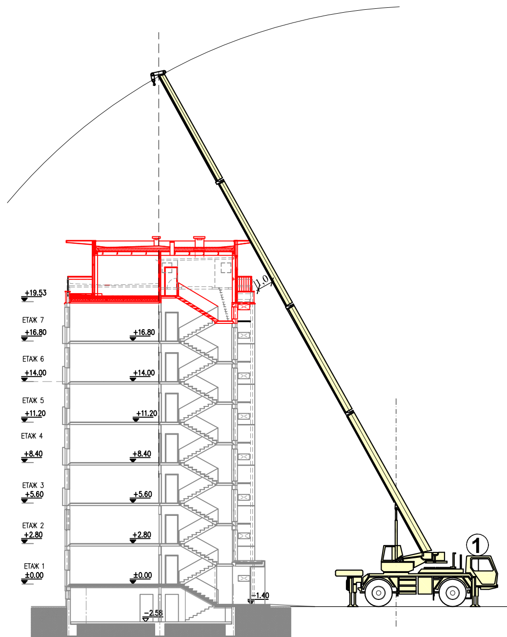
РАЗРЕЗ А-А
