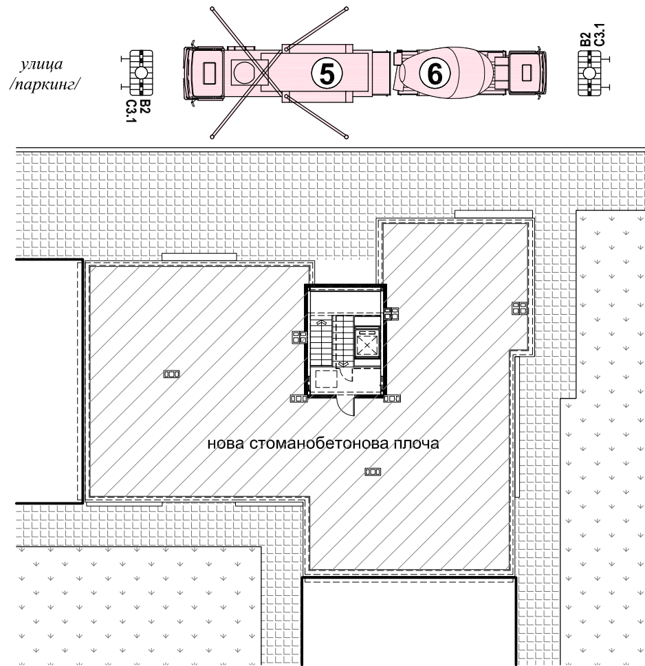
ПОКРИВ ВАРИАНТ С ДОЛИВАНЕ НА ПЛОЧА ЗА ДОСТЪП ДО ПОКРИВА
