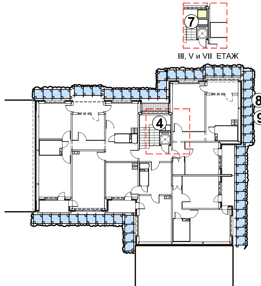
ТИПОВ ЕТАЖ
