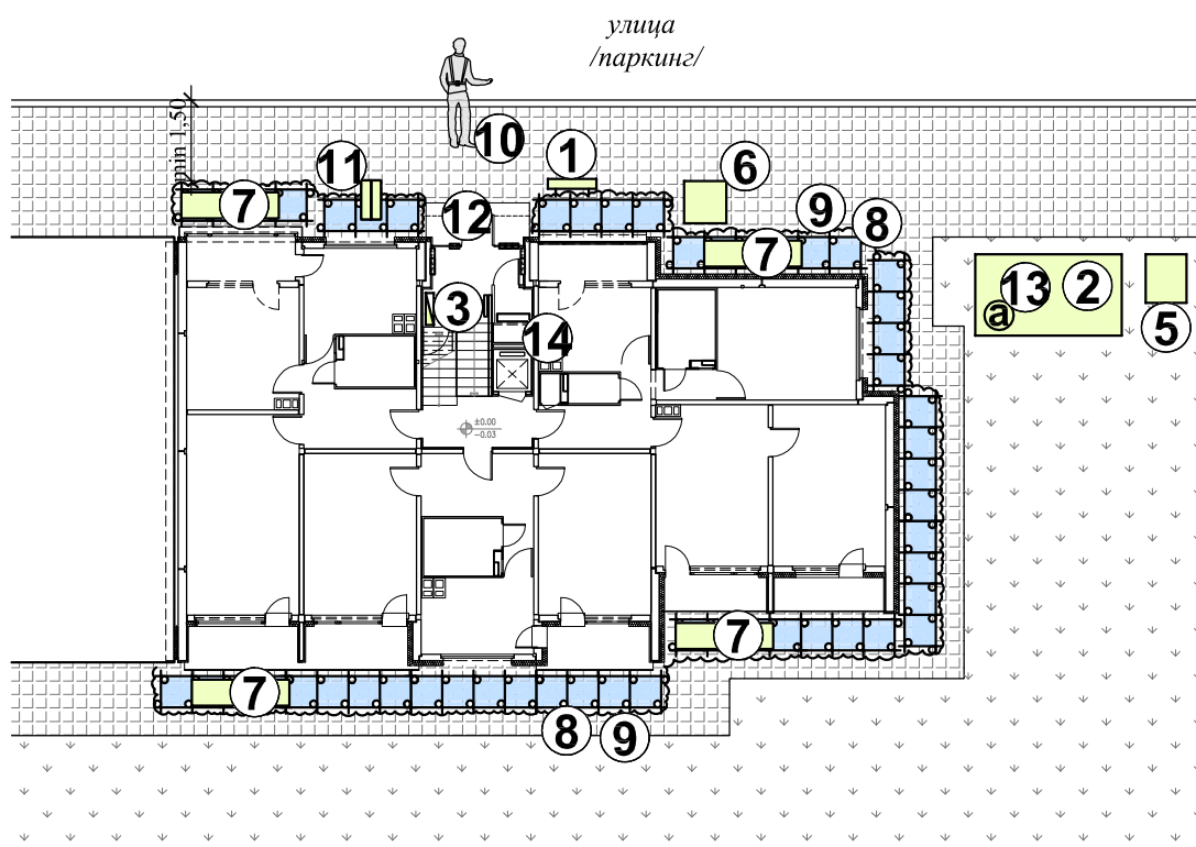
ПЪРВИ ЕТАЖ
