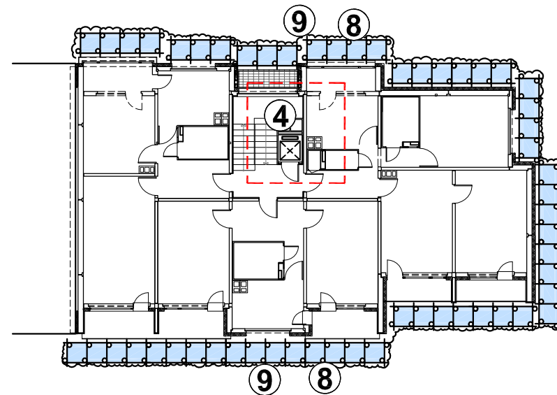
ТИПОВ ЕТАЖ
