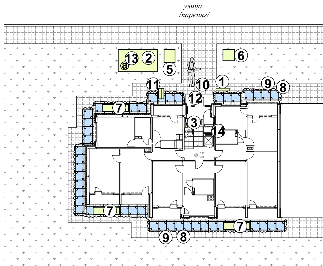
ПЪРВИ ЕТАЖ
