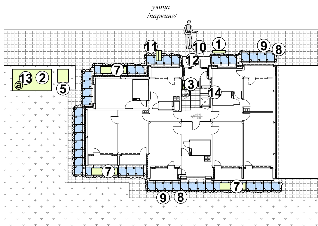
ПЪРВИ ЕТАЖ
