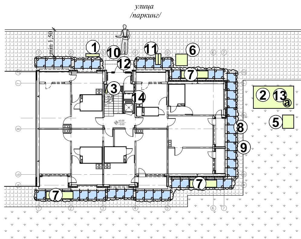
ПЪРВИ ЕТАЖ
