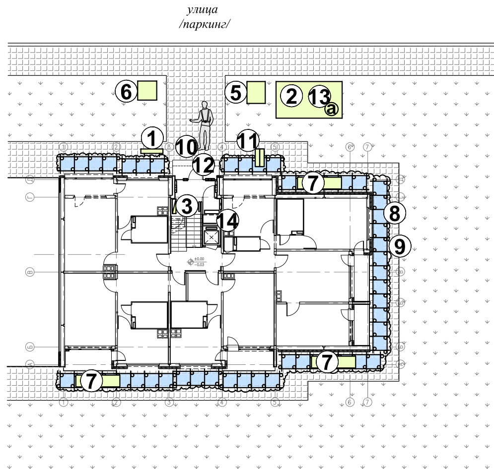
ПЪРВИ ЕТАЖ
