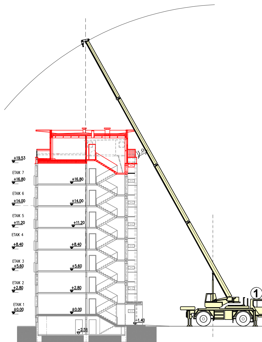
РАЗРЕЗ А-А
