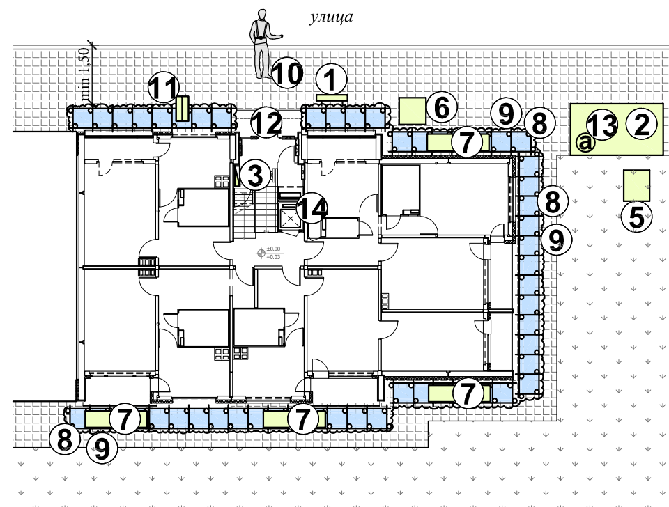
ПЪРВИ ЕТАЖ
