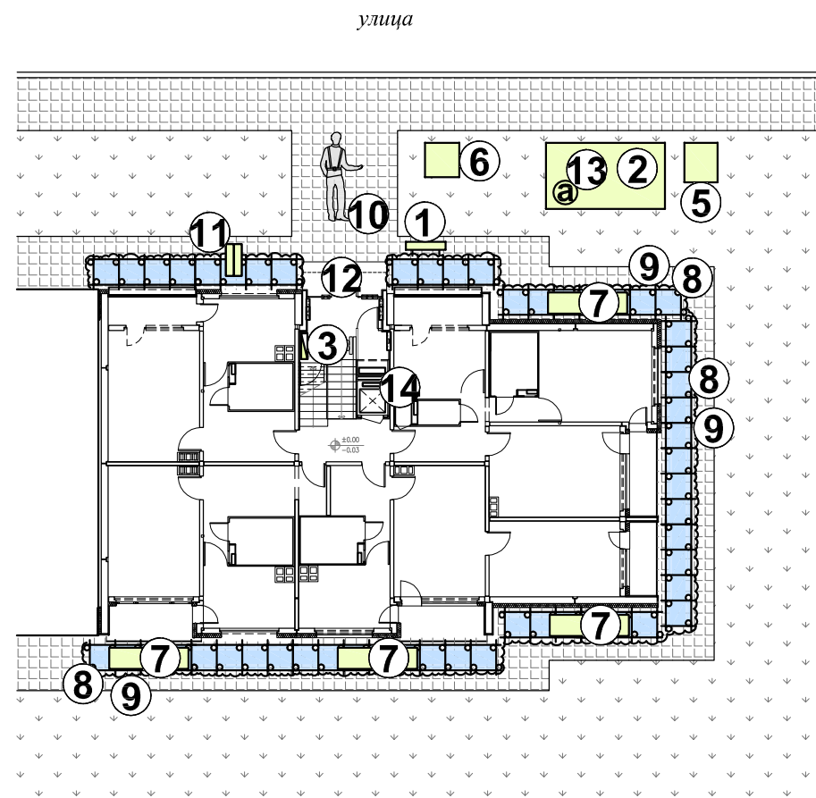
ПЪРВИ ЕТАЖ
