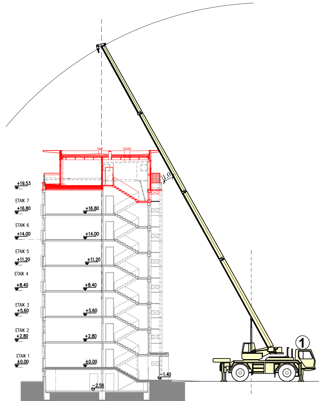
РАЗРЕЗ А-А
