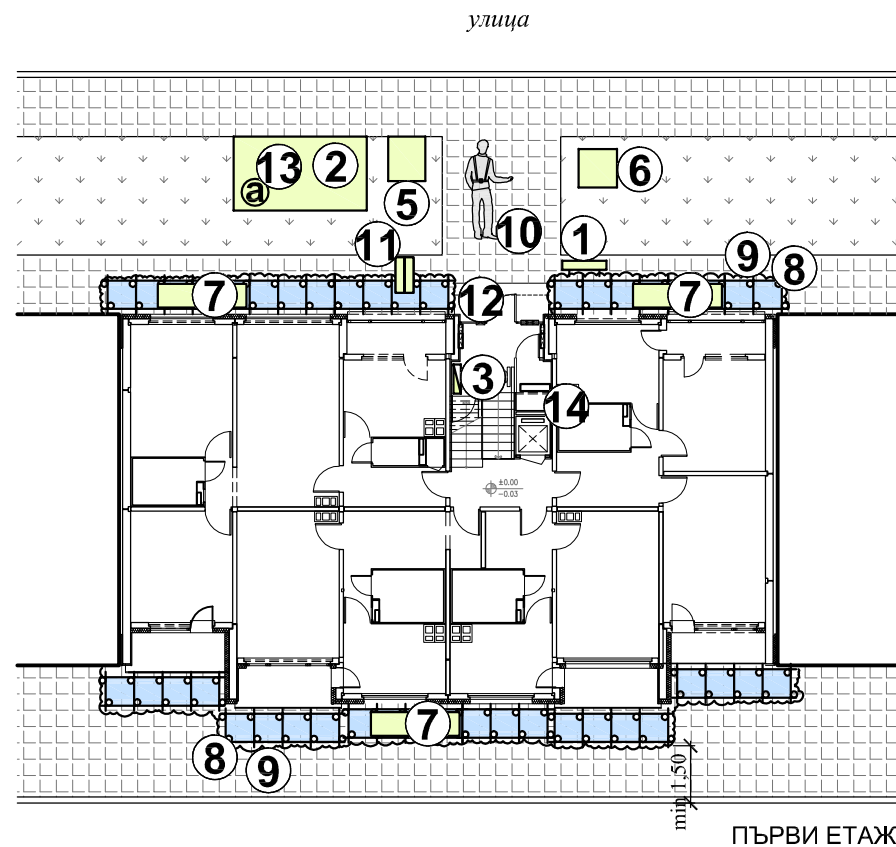
ВАРИАНТ ДВЕ УЛИЦИ
