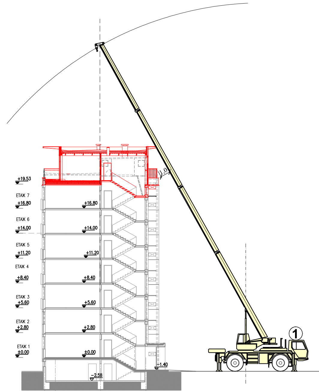
РАЗРЕЗ А-А
