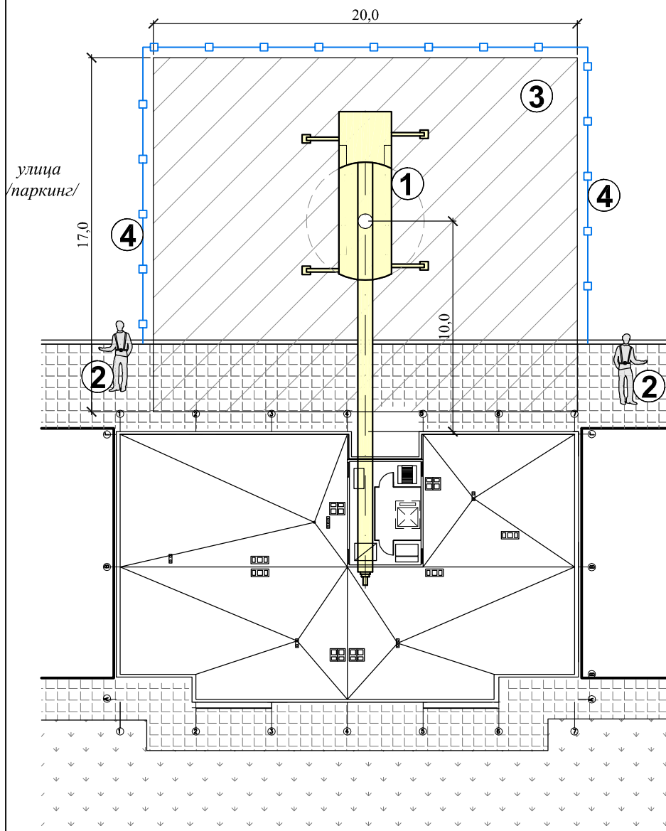
СЪЩЕСТВУВАЩ ПОКРИВ ДЕМОНТАЖ НА ПОКРИВНИ ПАНЕЛИ; МОНТАЖ НА ПАНЕЛИ ТИП "СПИРОЛ" ЗА ДОСТЪП ДО ПОКРИВА
