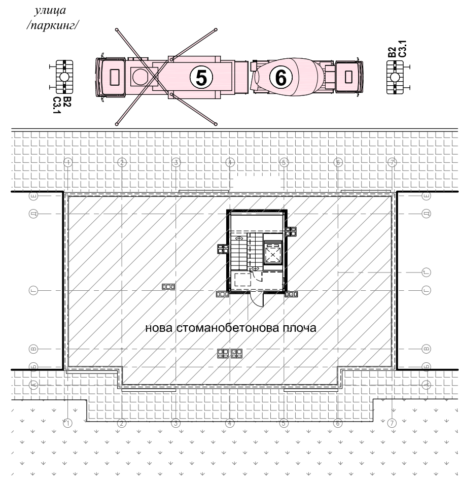
ПОВИВ ВАРИАНТ С ДОЛИВАНЕ НА ПЛОЧА ЗА ДОСТЪП ДО ПОКРИВА
