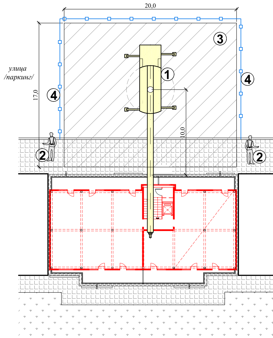
НАДСТРОЙКА МОНТАЖ НА ПАНЕЛИ ТИП "СПИРОЛ" И МЕТАЛНИ КОНСТРУКЦИИ
