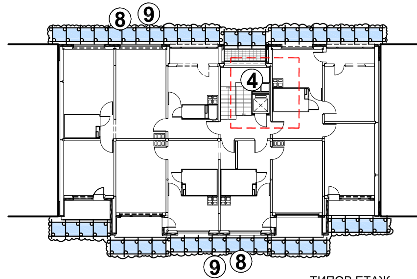
ТИПОВ ЕТАЖ
