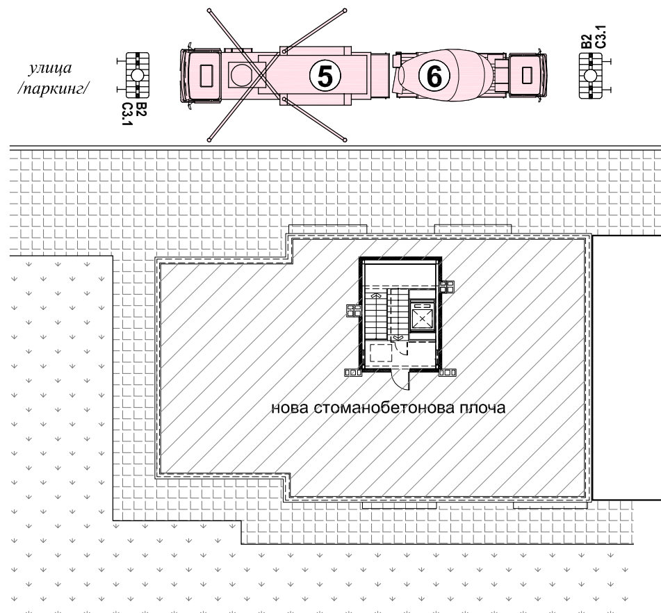
ПОКРИВ ВАРИАНТ С ДОЛИВАНЕ НА ПЛОЧА ЗА ДОСТЪП ДО ПОКРИВА
