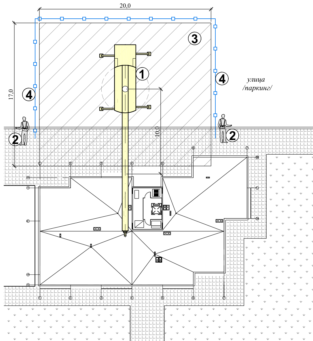
СЪЩЕСТВУВАЩ ПОКРИВ ДЕМОНТАЖ НА ПОКРИВНИ ПАНЕЛИ; МОНТАЖ НА ПАНЕЛИ ТИП "СПИРОЛ" ЗА ДОСТЪП ДО ПОКРИВА
