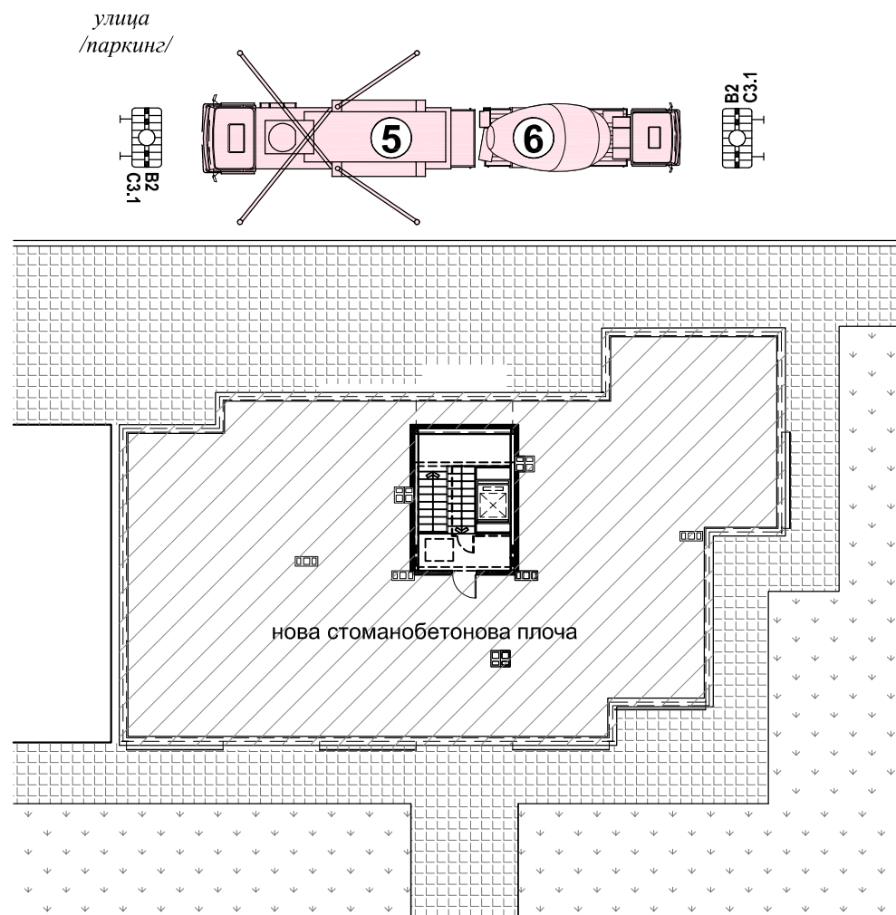
ПОКРИВ ВАРИАНТ С ДОЛИВАНЕ НА ПЛОЧА ЗА ДОСТЪП ДО ПОКРИВА
