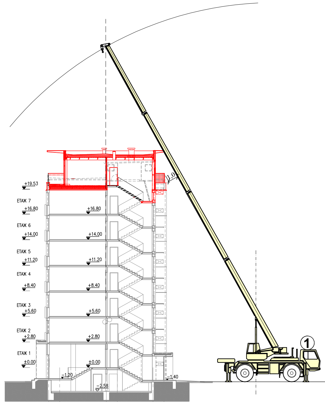
РАЗРЕЗ А-А
