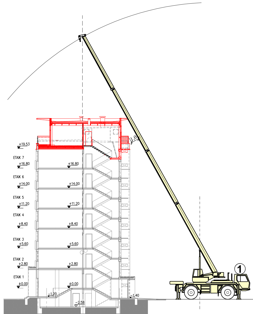
РАЗРЕЗ А-А
