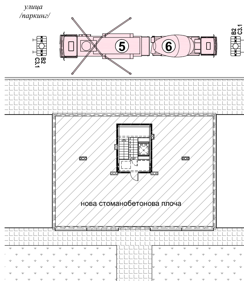
ПОКРИВ ВАРИАНТ С ДОЛИВАНЕ НА ПЛОЧА ЗА ДОСТЪП ДО ПОКРИВА
