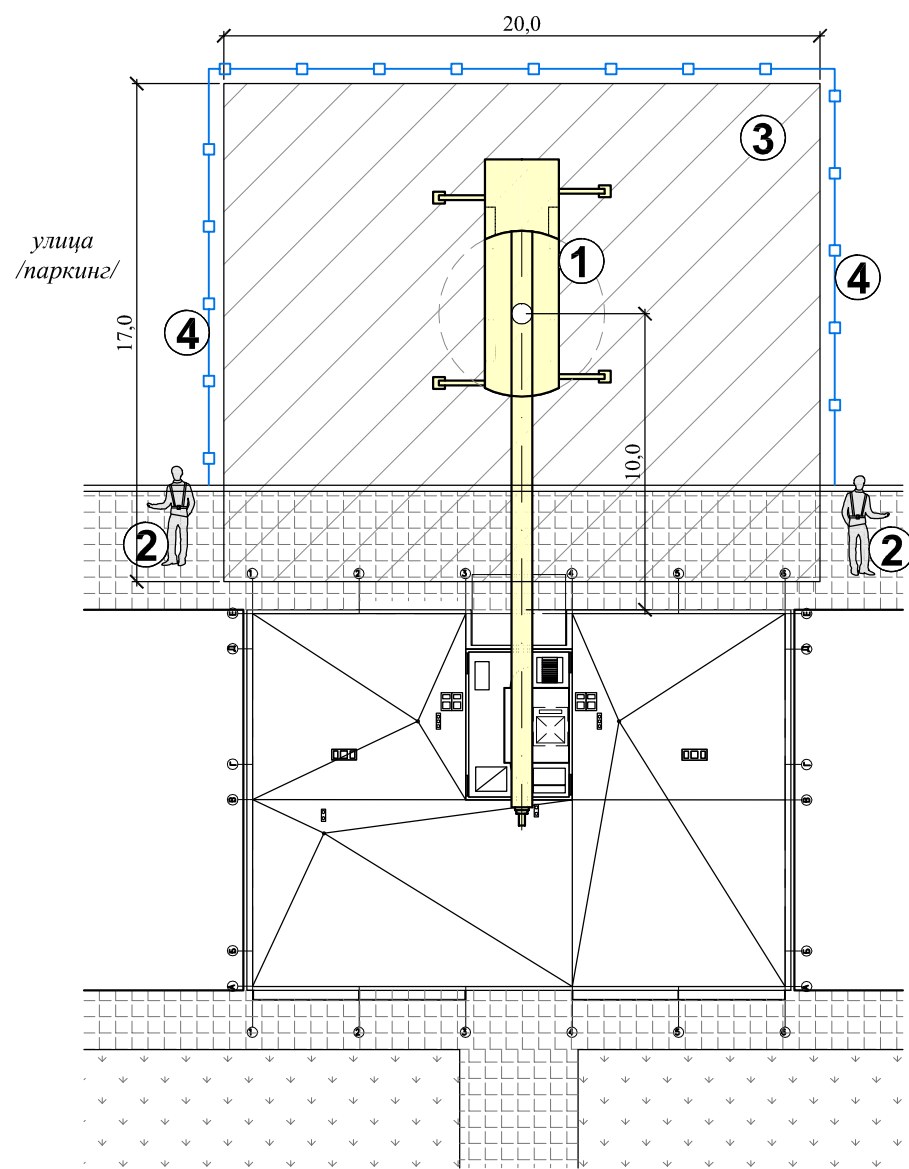
СЪЩЕСТВУВАЩ ПОКРИВ ДЕМОНТАЖ НА ПОКРИВНИ ПАНЕЛИ; МОНТАЖ НА ПАНЕЛИ ТИП "СПИРОЛ" ЗА ДОСТЪП ДО ПОКРИВА
