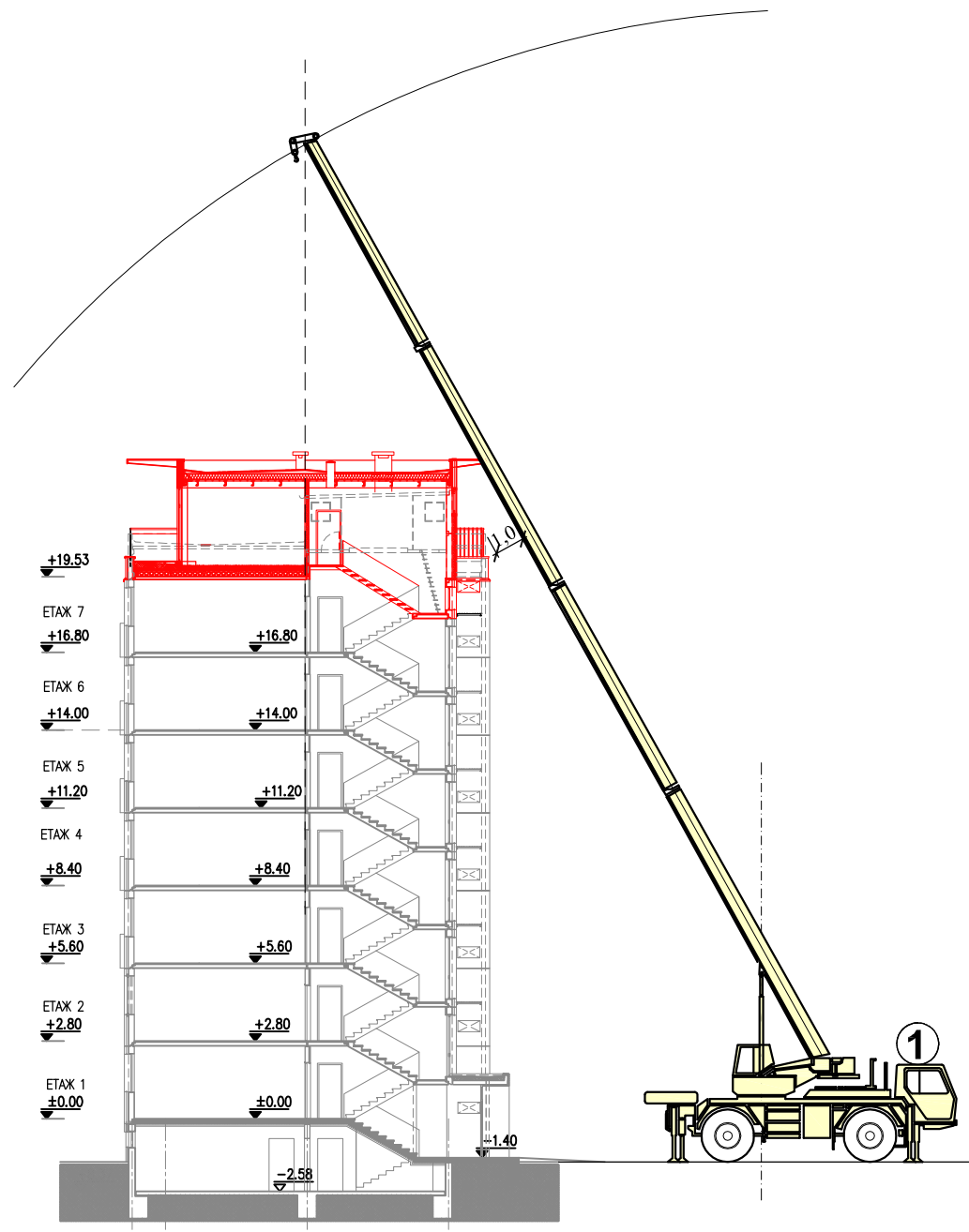
РАЗРЕЗ А-А
