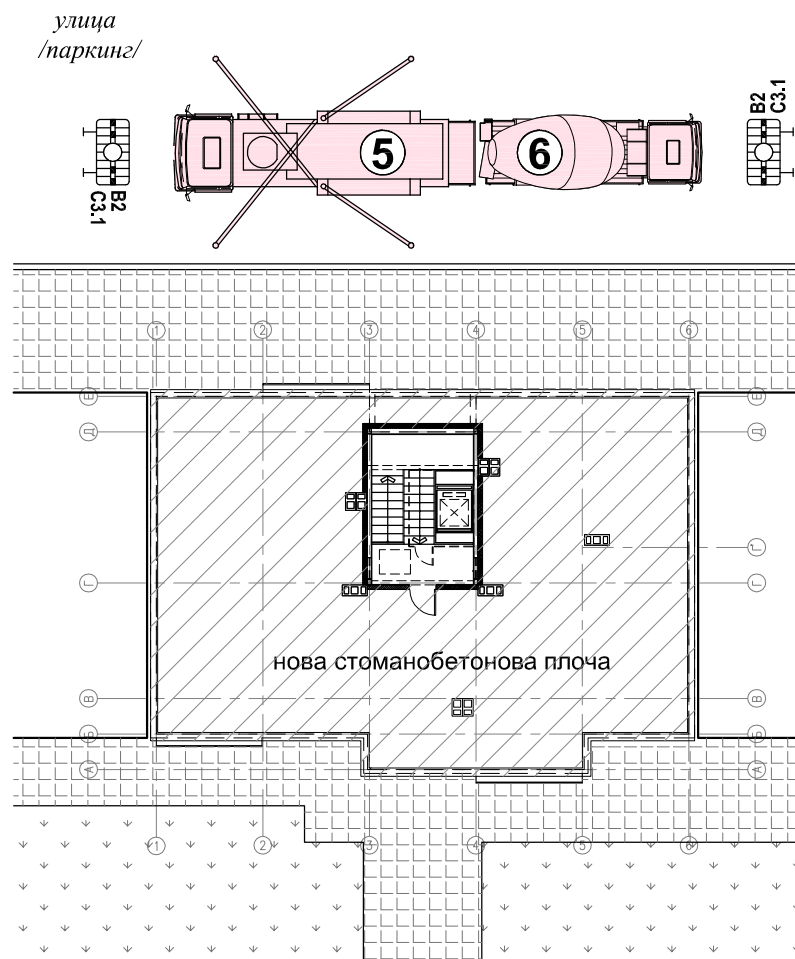
ПОКРИВ ВАРИАНТ С ДОЛИВАНЕ НА ПЛОЧА ЗА ДОСТЪП ДО ПОКРИВА
