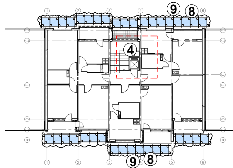
ТИПОВ ЕТАЖ
