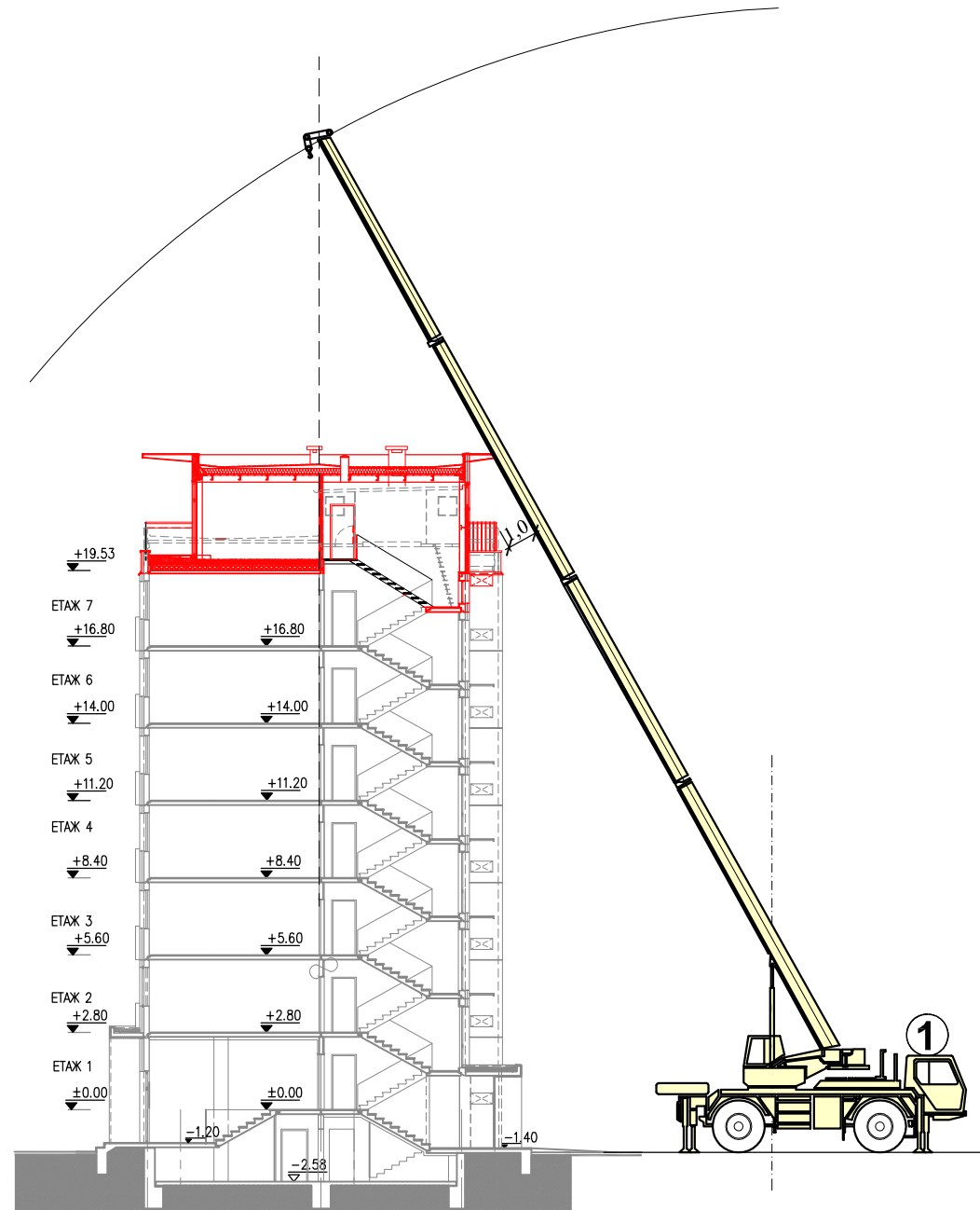
РАЗРЕЗ А-А
