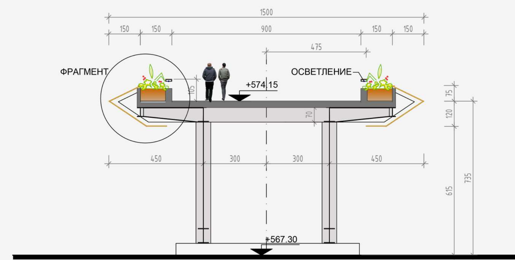
НАПРЕЧЕН РАЗРЕЗ - ЕСТАКАДА, М 1:100
