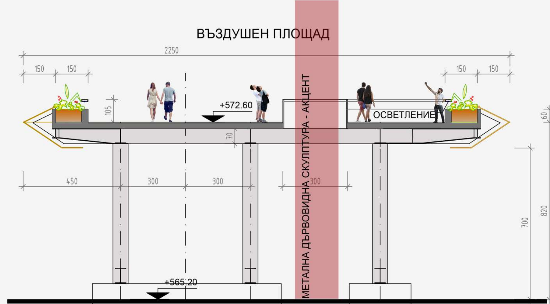
НАПРЕЧЕН РАЗРЕЗ ВЪЗДУШЕН ПЛОЩАД, М 1:100
